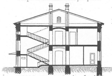
Разрѣзь пожарнаго здания по аб. Coupe de la maison des pompiers.
