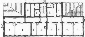
Планъ 1 го этажа арест зд. Maison d'arrêt, parterre
