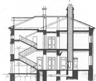
Разрѣзь арестнаго здания Maison d'arrêt Coupe
