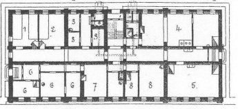
Планъ 1 го этажа арест зд. Maison d'arrêt, parterre
