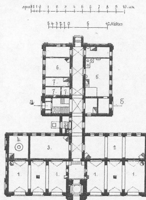
Планъ 1 го этажа пожар отд. Partier de la mais des pompiers.
