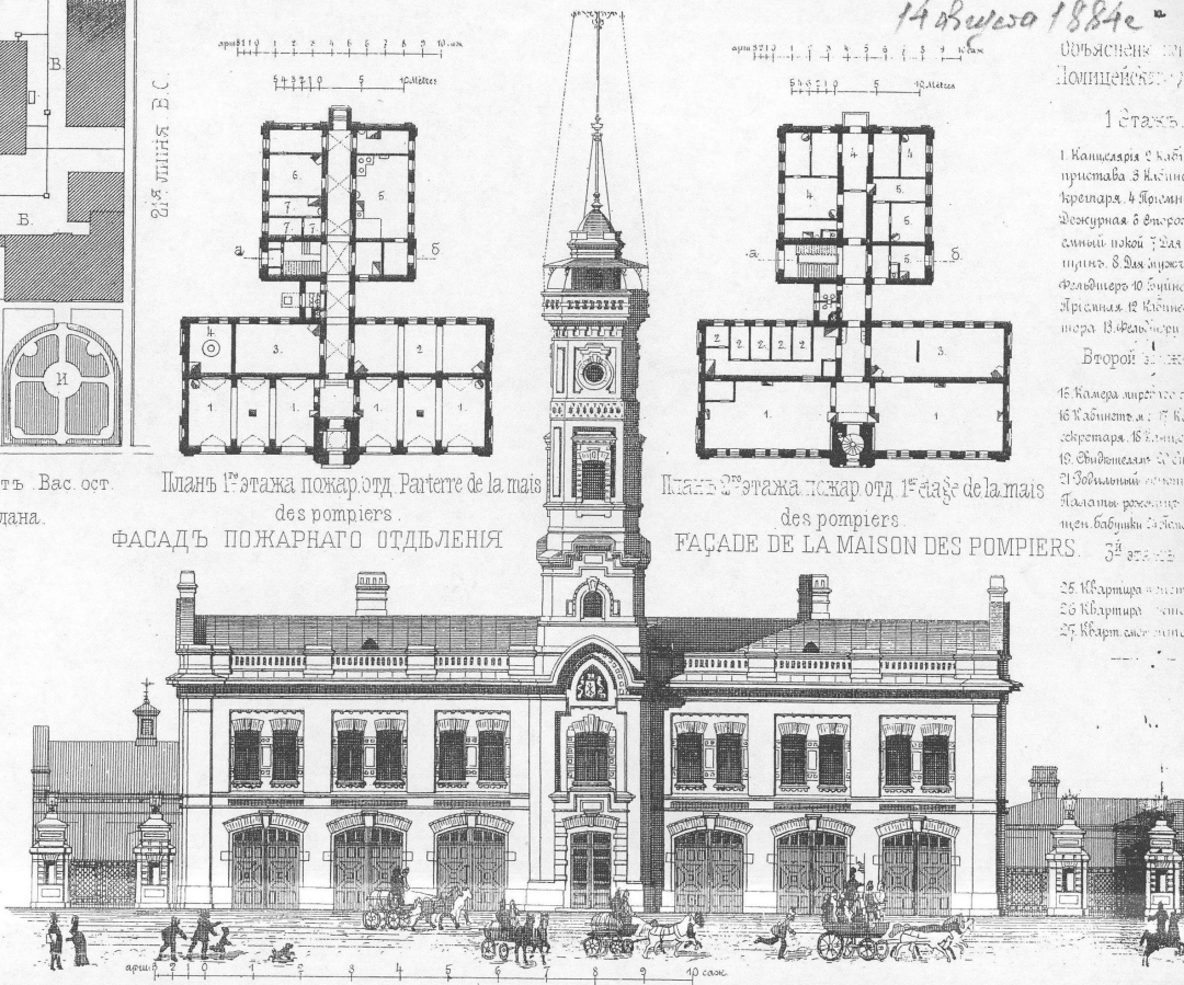
План здания Васильевской пожарной части
