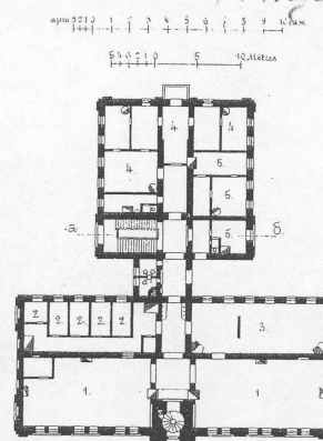
Планъ 2 го этажа пожар отд. 1 го étage de la mais des pompiers.
